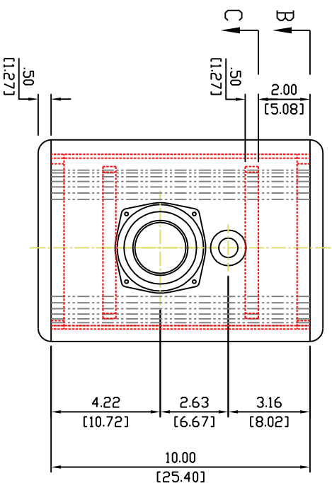
View A-A
